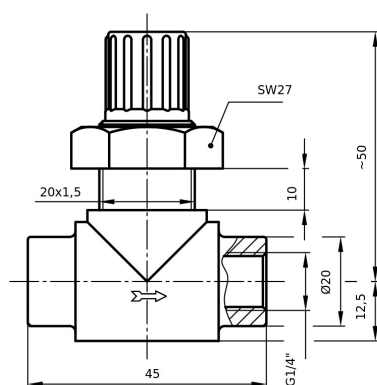
Chiffres en mm; Illustration à titre d'exemple
