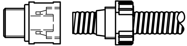
コネクタ本体 圧力ネジ コルゲートチューブ
